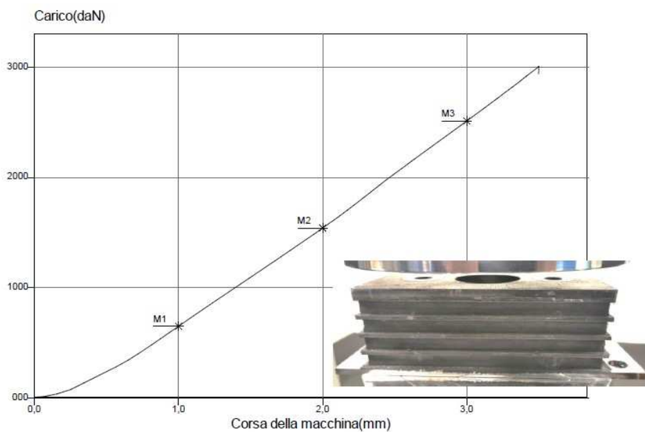
Test carico/cedimenti assiale su campione a durezza sh. 60
